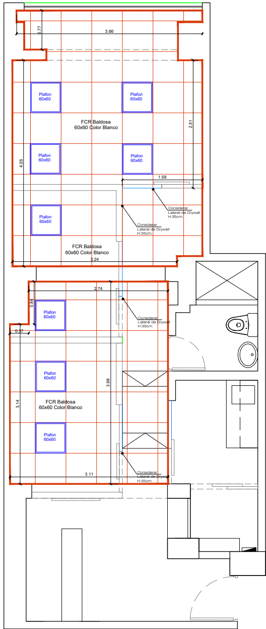
PRIMER PISO PLANO FALSO CIELO RASO + Esquema IIEE Esc 1:75
