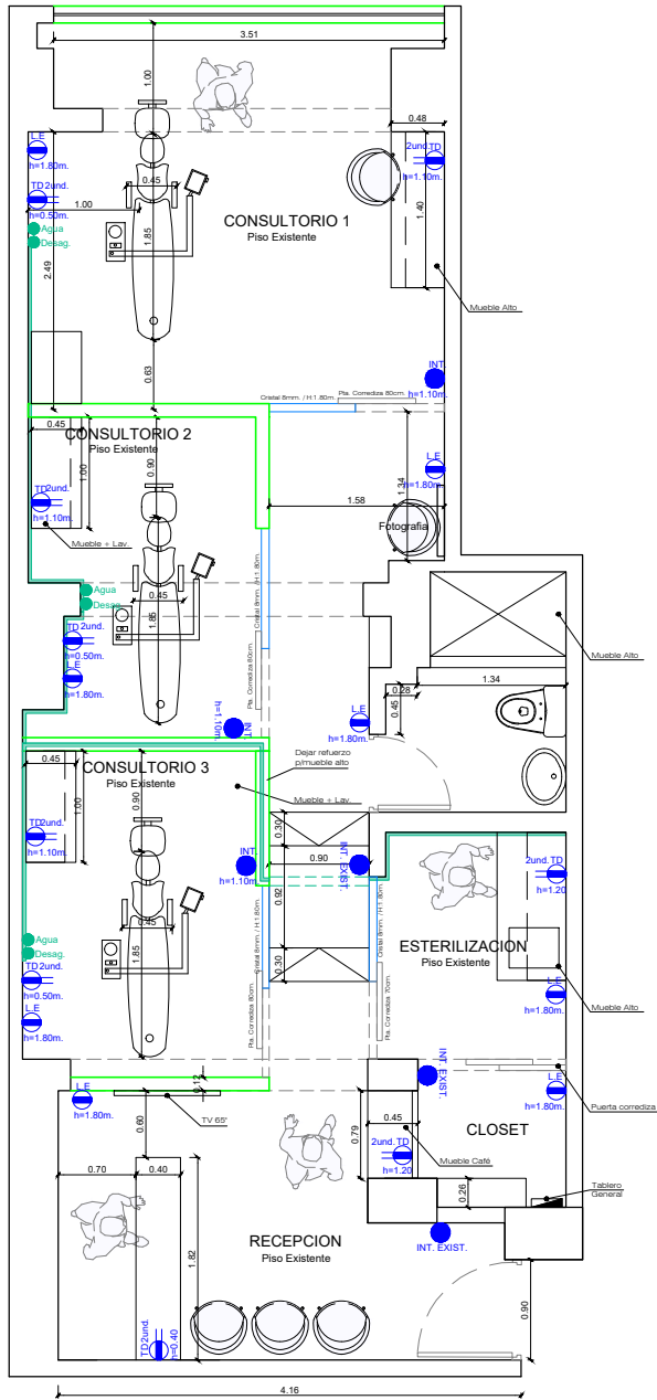
PRIMER PISO PLANO ARQ + Esquema IIEE // IISS Esc 1:75
